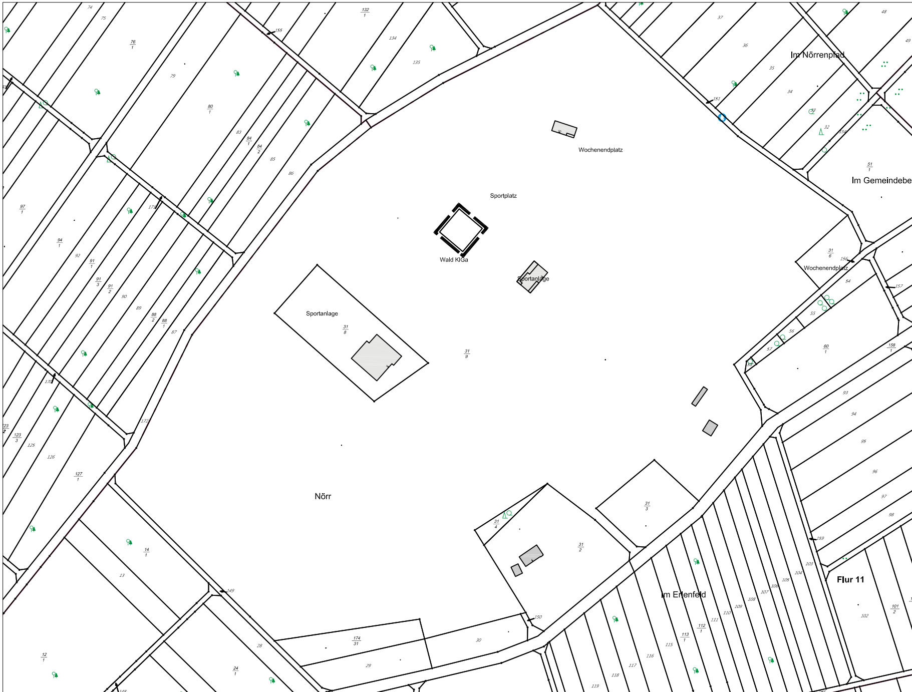
Übersichtsplan zur Ausstellung des Bebauungsplanes "Wald- und Naturkindergarten" der Ortsgemeinde Eitelborn
