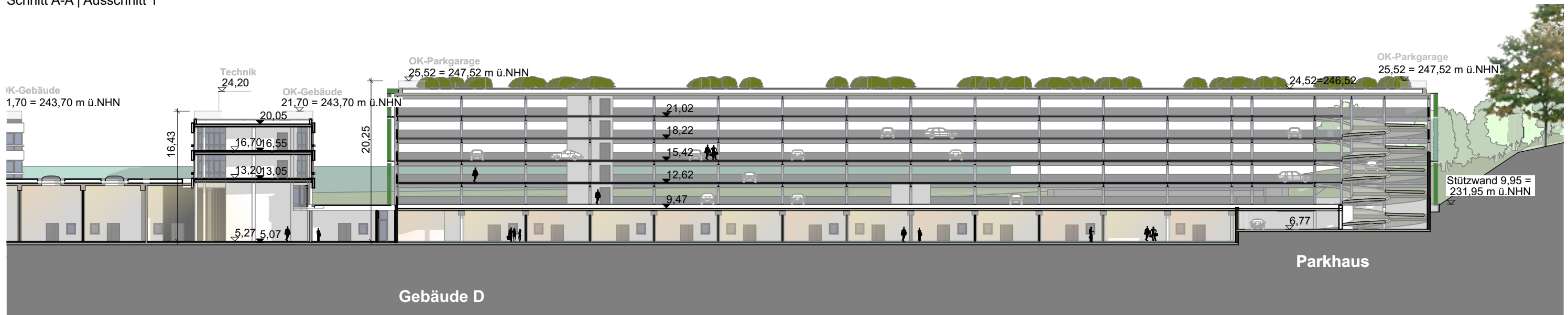
Schnitt A-A | Ausschnitt 2
