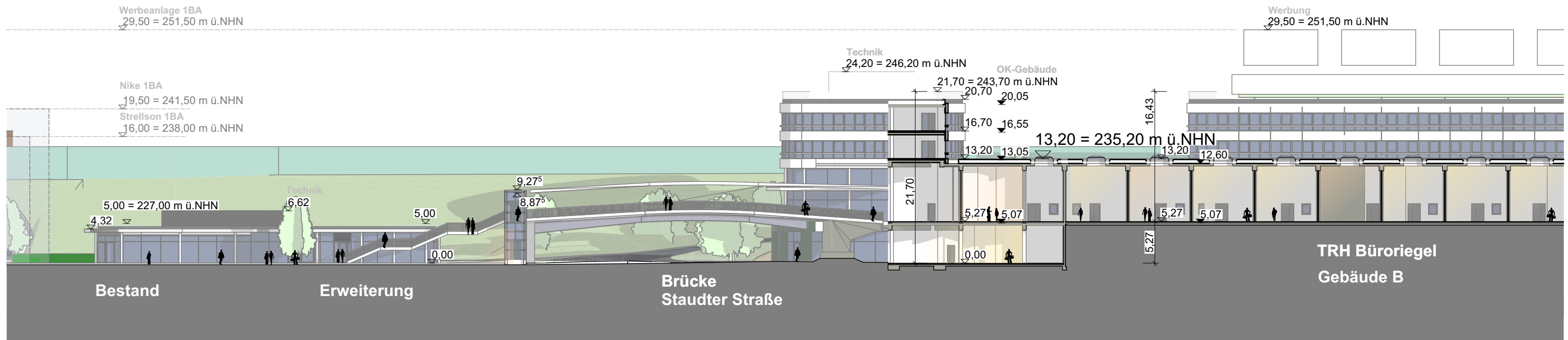
Schnitt A-A | Ausschnitt 1
