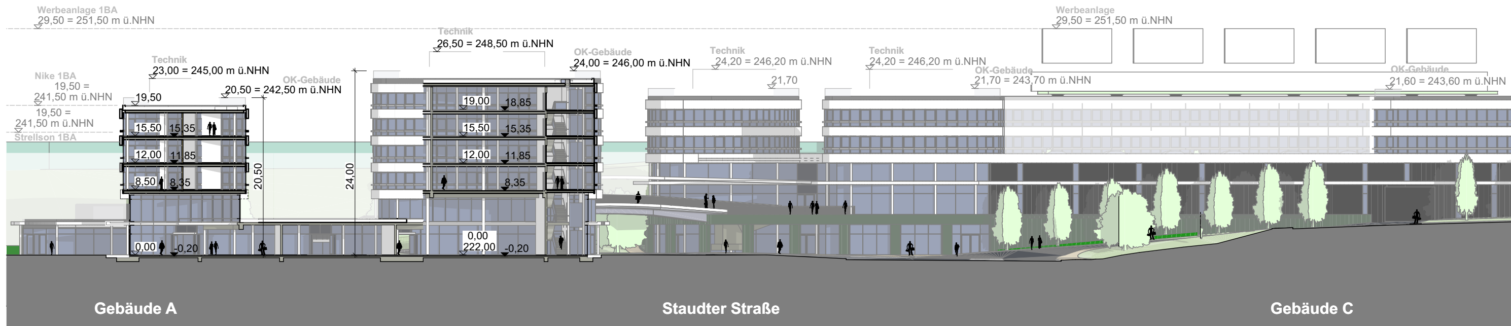
Schnitt B-B | Ausschnitt 1
